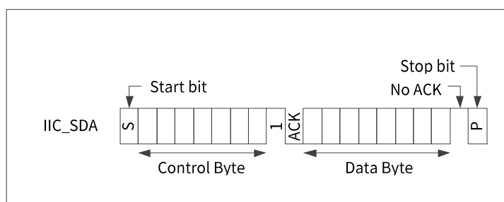
图27. I 2 C 随机读取格式
