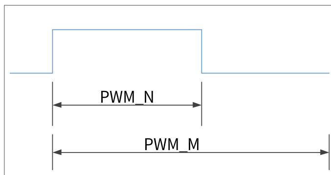
图19. PWM 时序设置图
