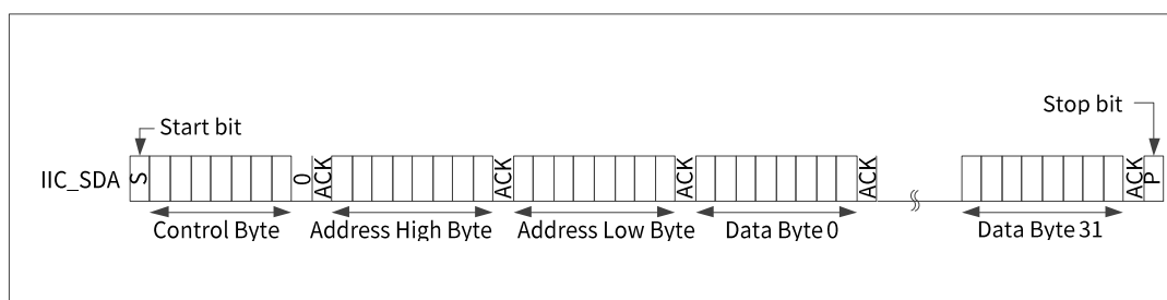
图26. I 2 C 当前读取格式
