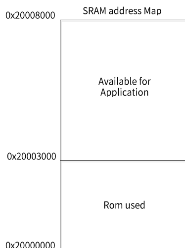
图13. Data SRAM 地址映射
