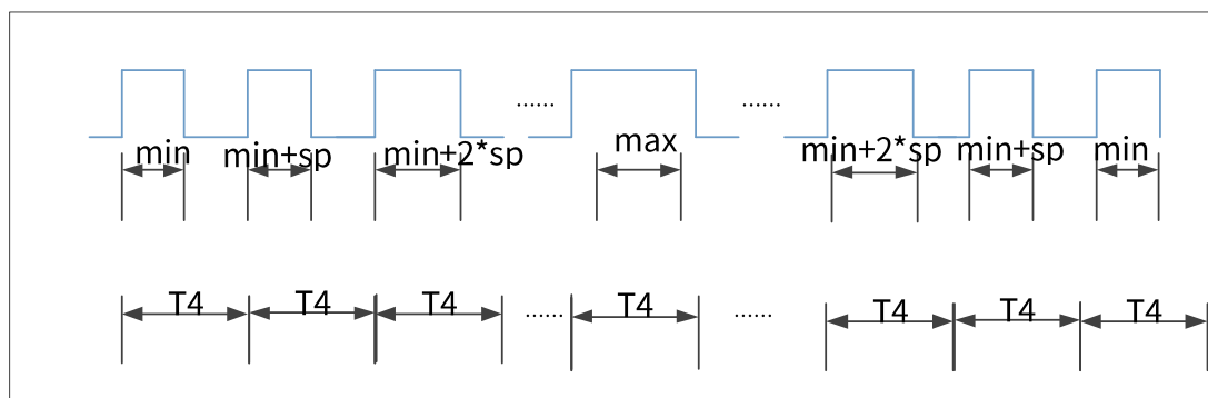
图21. LED呼吸灯设置图
