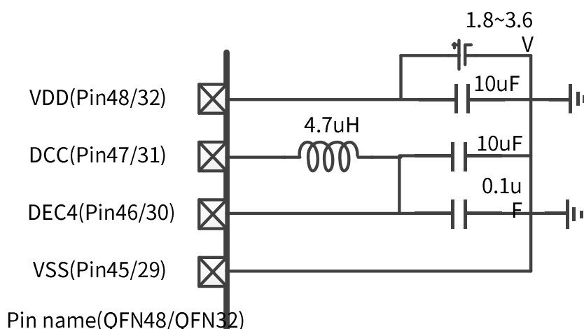
图15. DCDC 降压转换器配置
