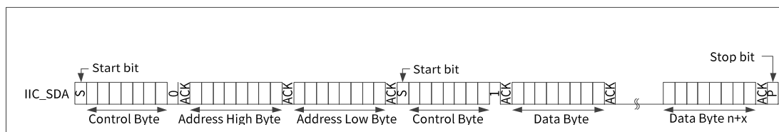
图28. I 2 C 顺序读取格式
