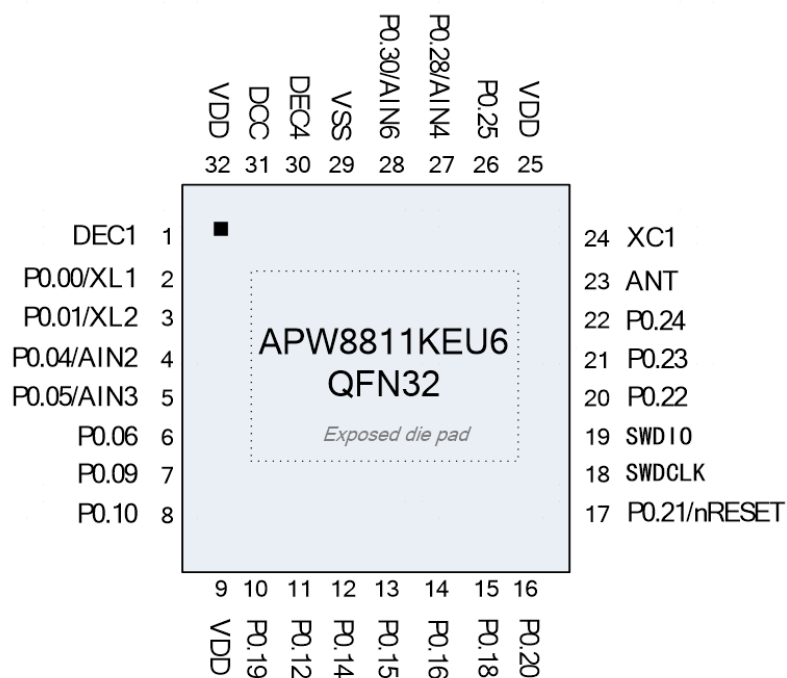
图2. QFN32 封装管脚定义(5mm*5mm)
