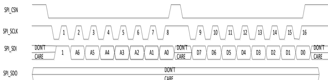
图30. 4-线 SPI 写操作
