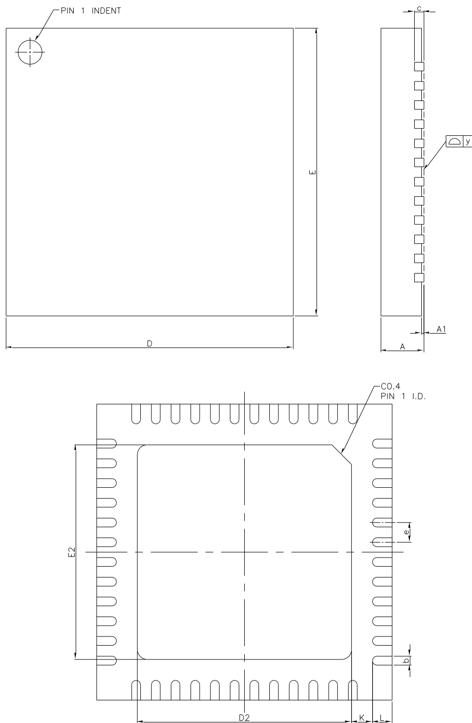
图11. APW8811CEU6 封装轮廓图和尺寸
