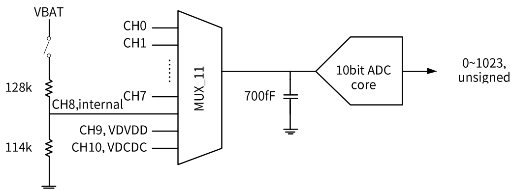
图14. GPADC 输入通道选择和电阻分压器配置
