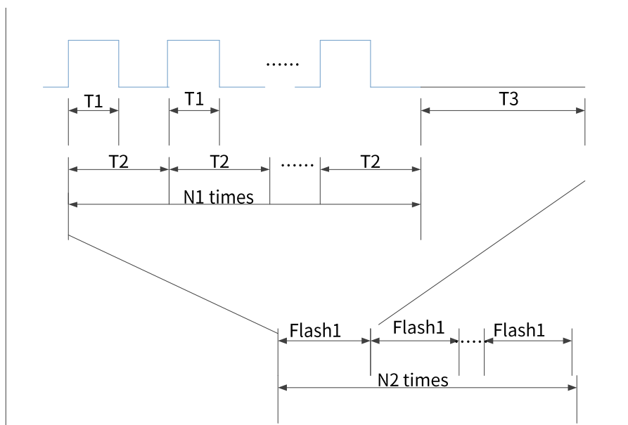
图20. LED 开-关设置图
