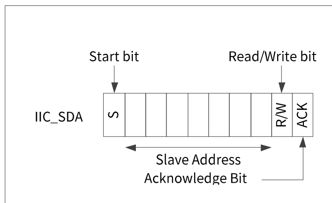
图24. I 2 C 字节写入格式
