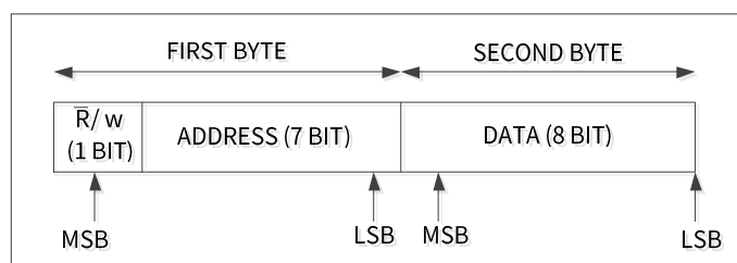
图29. 4 线 or 3/2-线 SPI 传输协议
