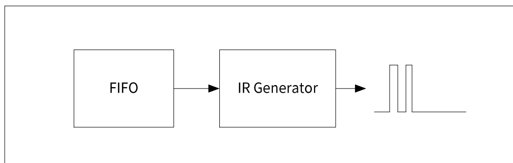
图37. IR 发生器功能框图
