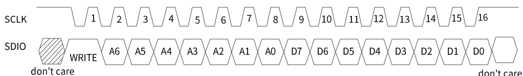
图31. 3/2-线 SPI 写操作
