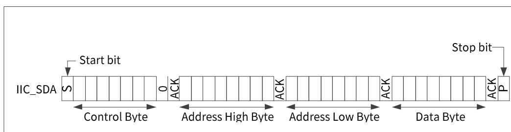
图25. I 2 C 页入格式
