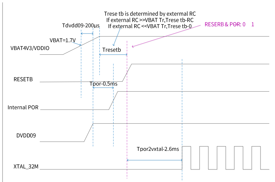
图4. 上电顺序
