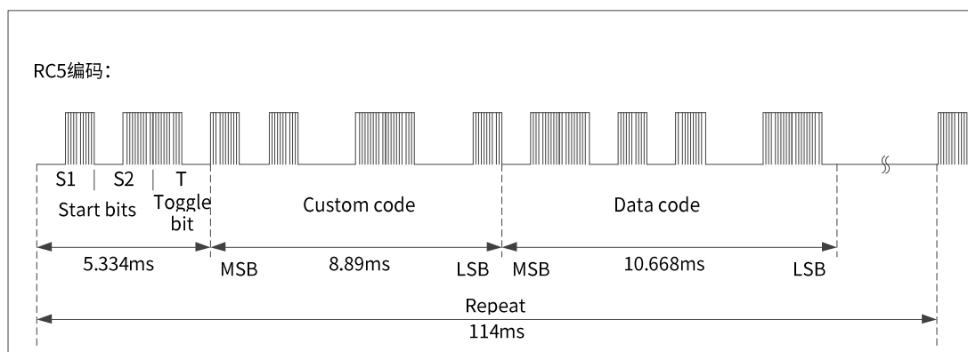
图39. RC5 编码波形格式
