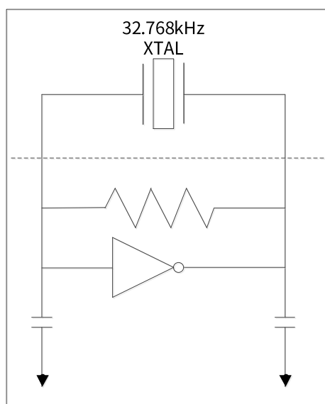
图6. 32.768KHz 晶体振荡器电路
