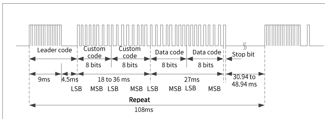
图38. NEC 编码波形格式
