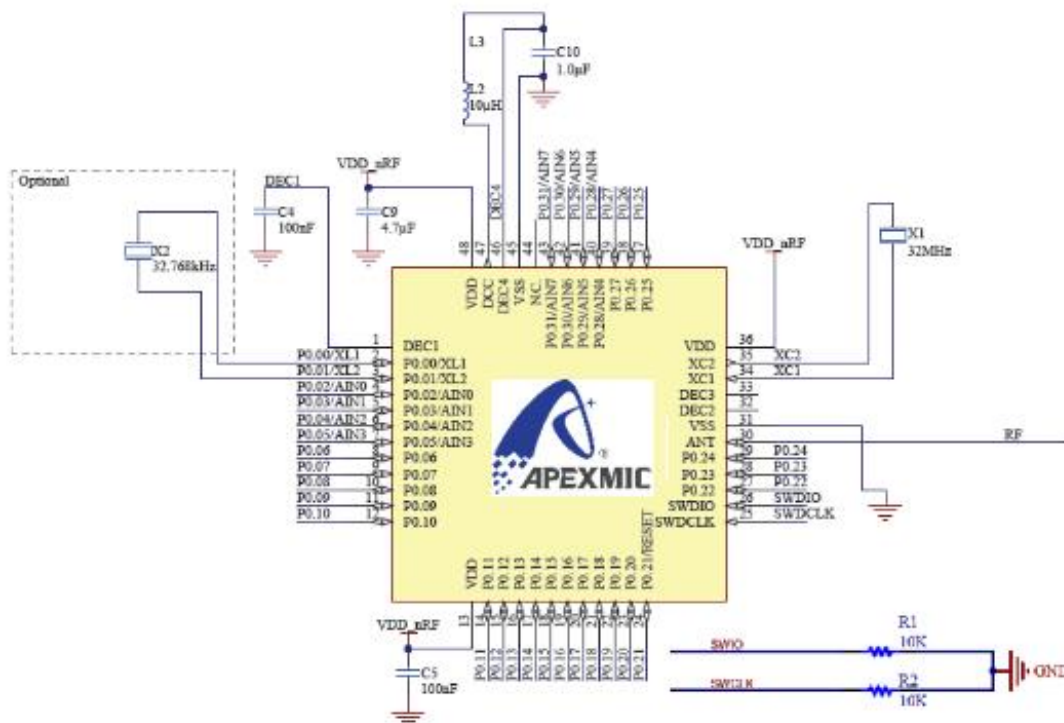
图8. APW8811CEU6 参考应用电路 (32.768K 晶振可选)
